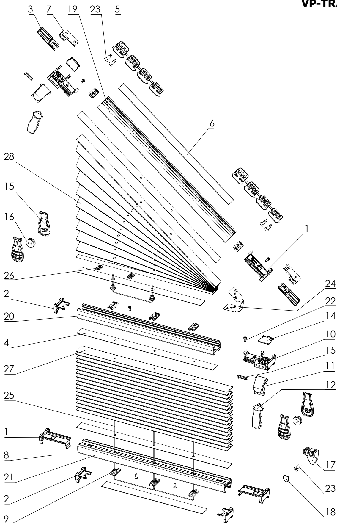
Schemat i wykaz elementów Vegas Plisse (trapez, obsługa sznurkiem, trzy profile)
